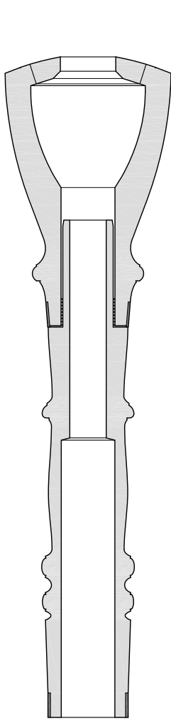
Sección da copa do roncón
