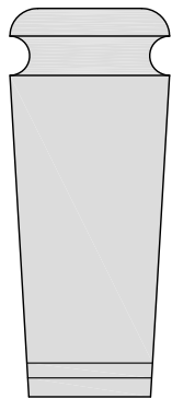
Vista da buxa do roncón
