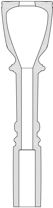
Sección da copa do roncón
