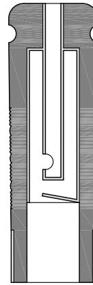
Sección
