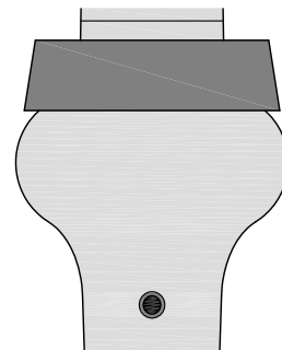
Detalle 2: anel de chapa de latón esp. 0,50 mm en furado do 1º grao superior - Escala 1 / 1
