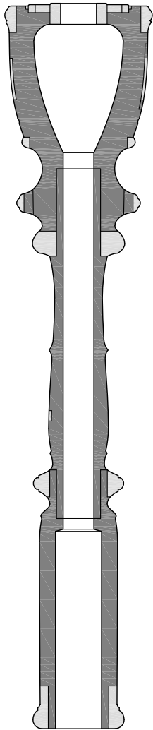
Sección da copa do roncón
