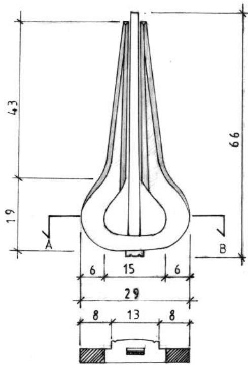
SECCION A:B
